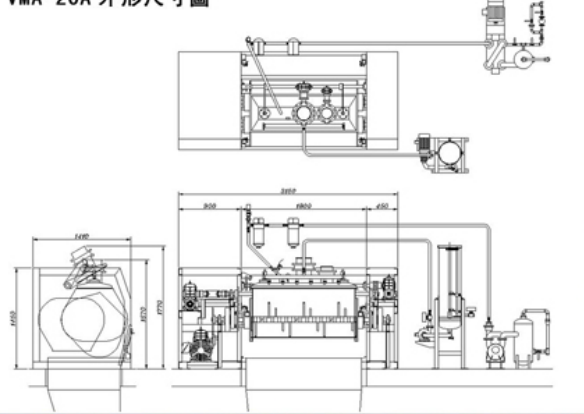
VMA-20A 外形尺寸圖
